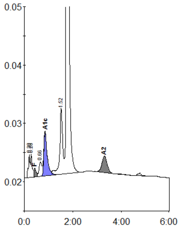
Peak table - ID: 2506025898
