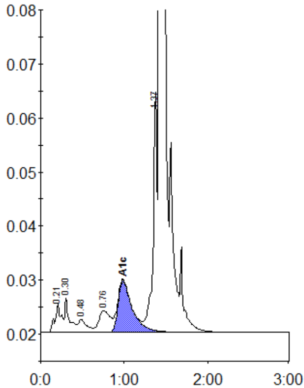
Peak table - ID: 10289091
