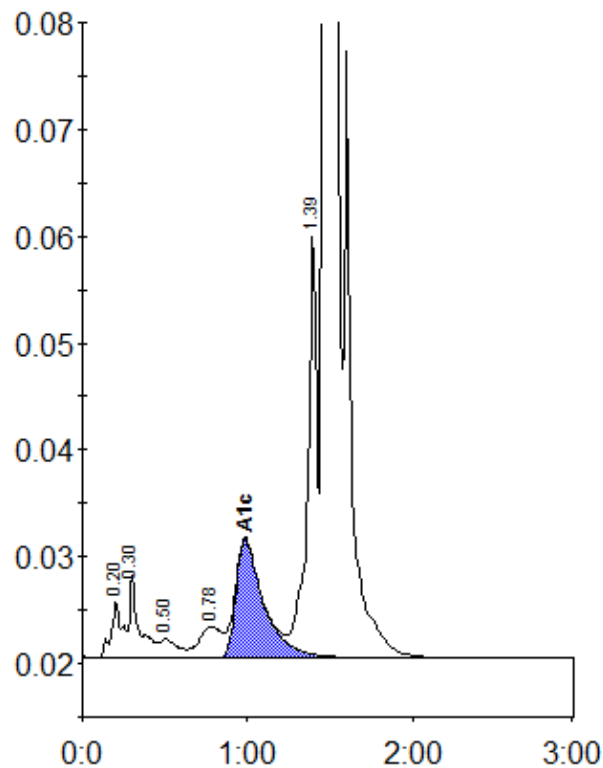
Peak table - ID: 10349676
