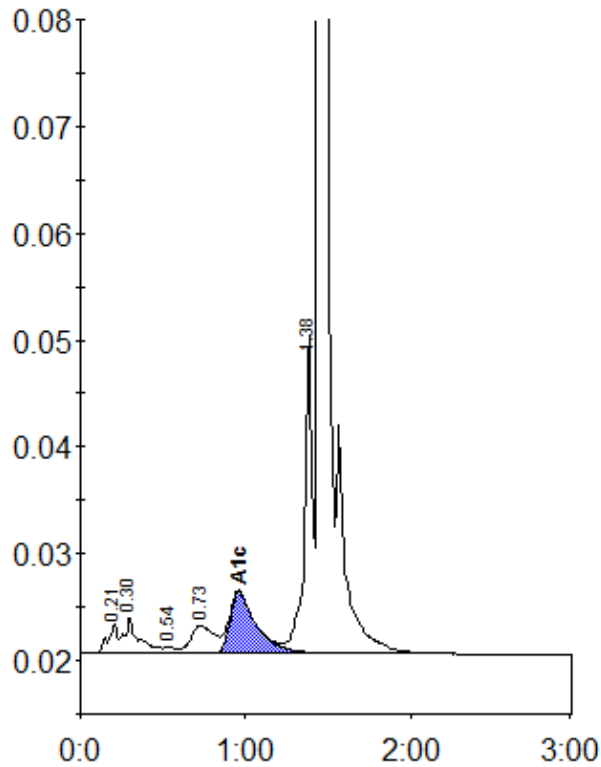
Peak table - ID: 10238888
