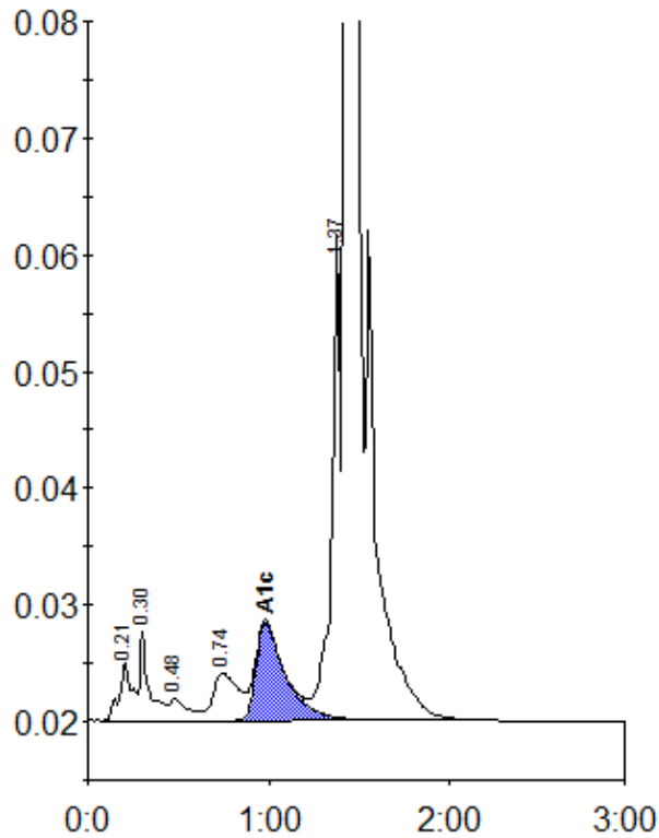
Peak table - ID: 10300178
