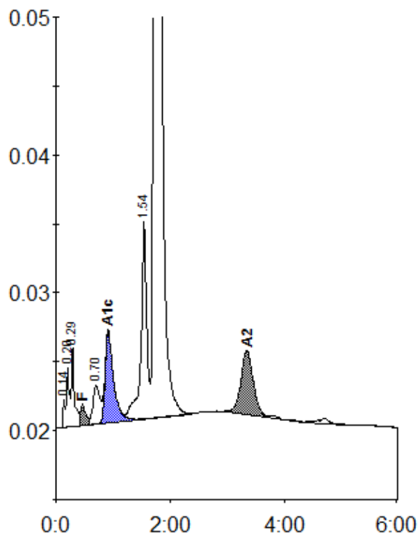
Peak table - ID: 10237624
