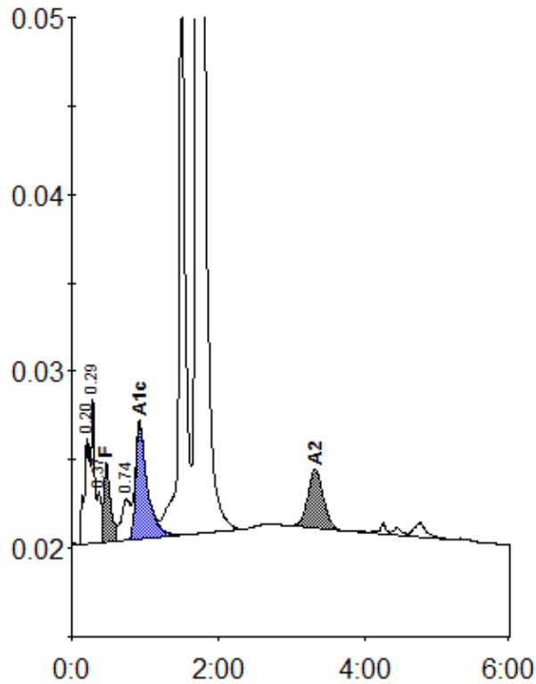
Peak table - ID: 10251430
