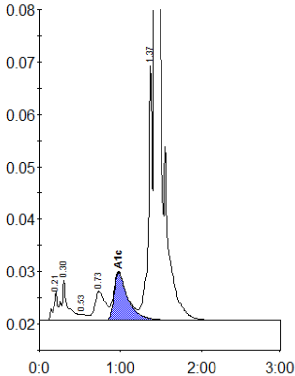
Peak table - ID: 10248962
