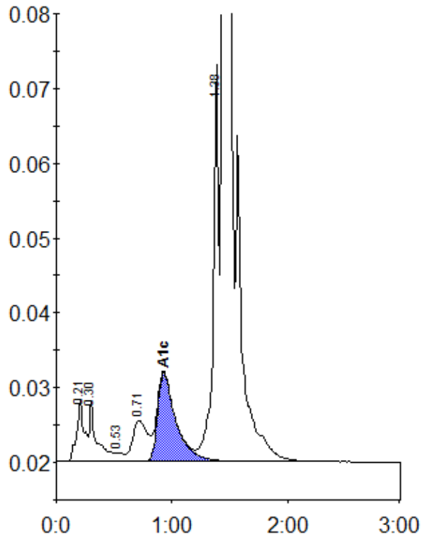
Peak table - ID: 10208204
