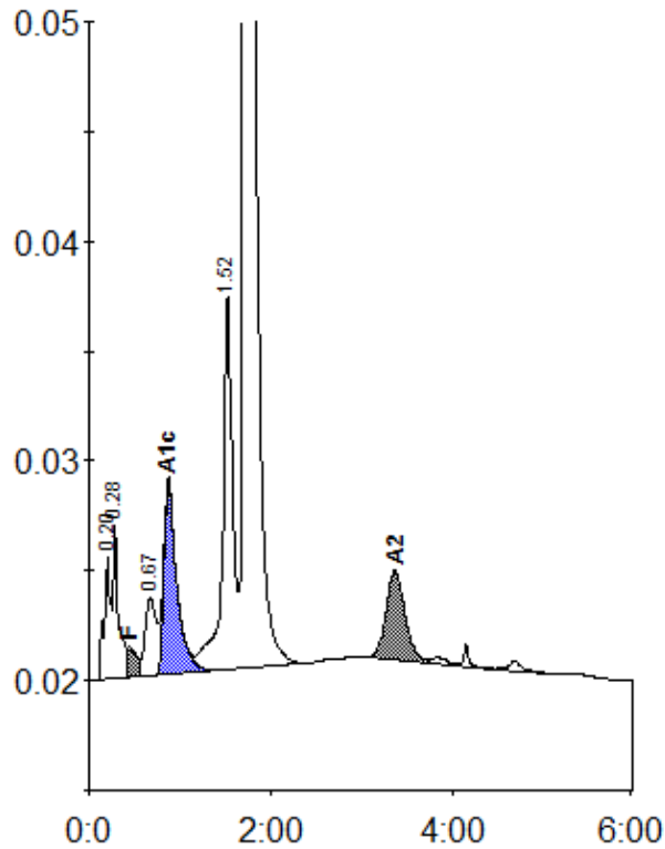
Peak table - ID: 10174233
