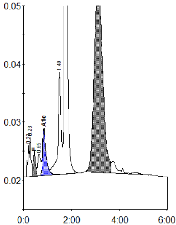
Peak table - ID: 10166804
