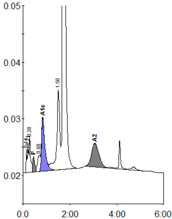
Peak table - ID: 10096736
