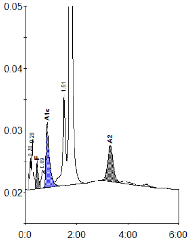
Peak table - ID: 10062695
